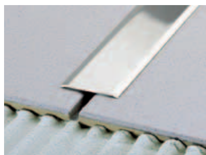
760/A_leštěná nerez ocel
